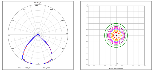
90° Reflector
